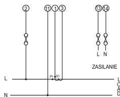
UKŁAD 1-FAZOWY
